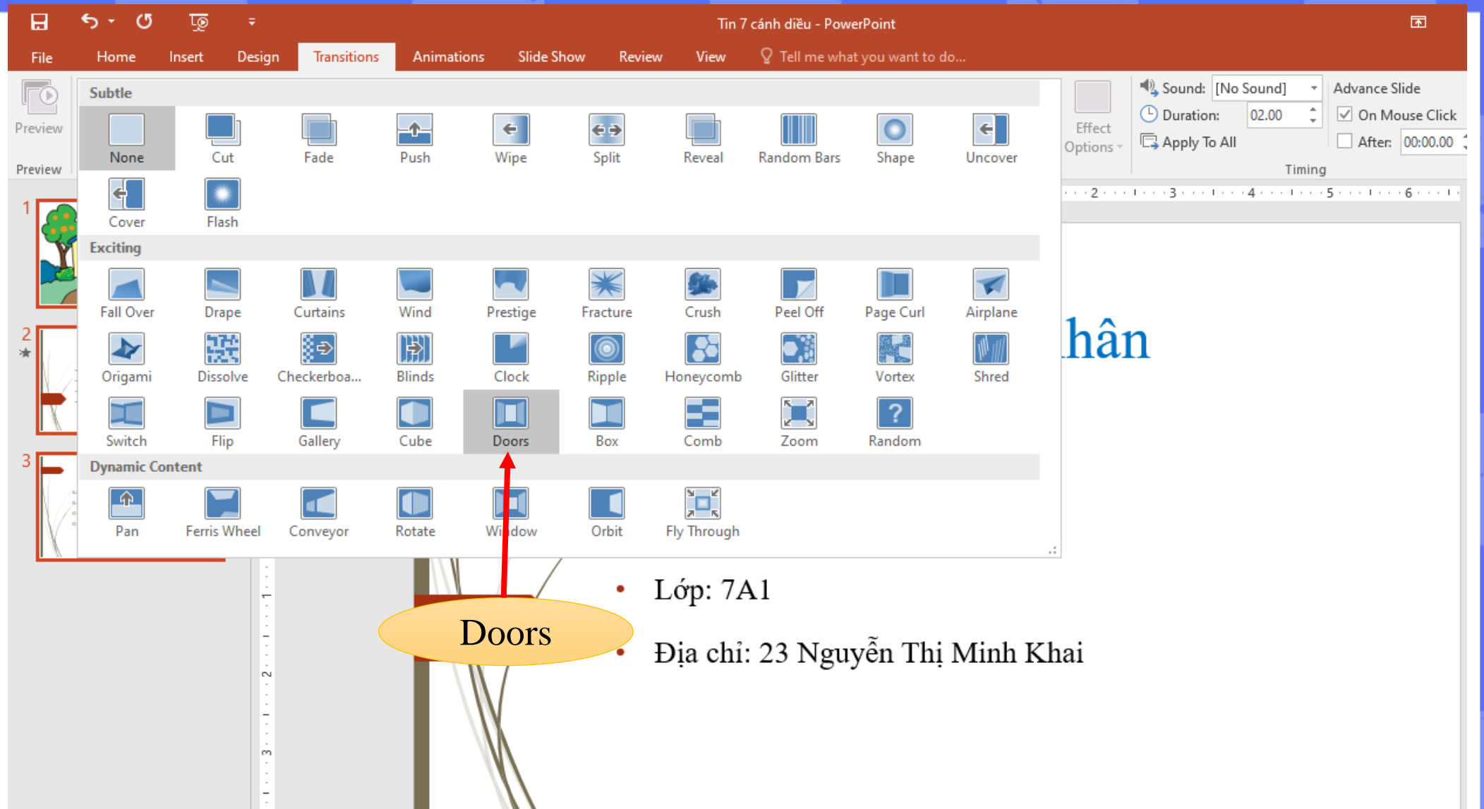
Hình 5. Chọn hiệu ứng Doors cho chuyển trang chiều
